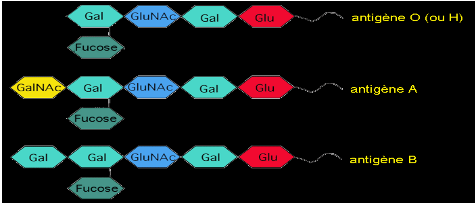
Structure glycanique des Antigènes ABO
