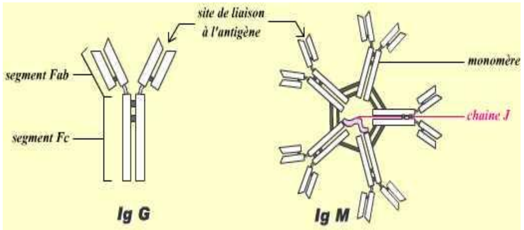
Schéma d'une immunoglobuline G et M
