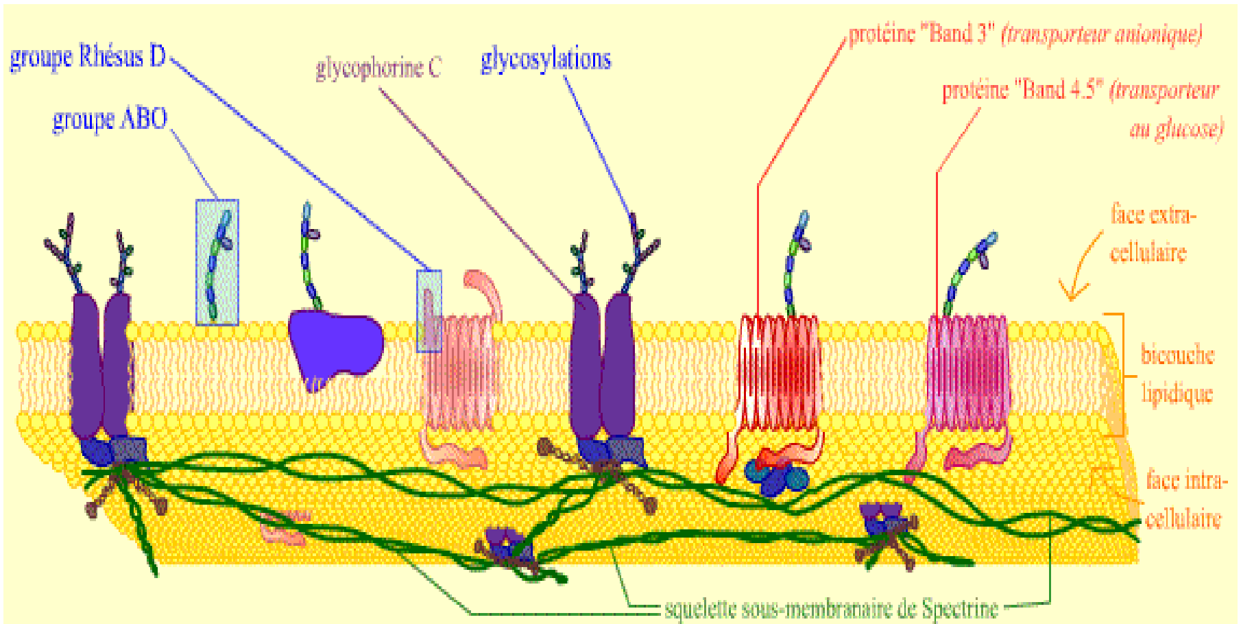
Représentation schématique de la membrane d'une hématie
